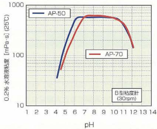
図2 水溶液粘度へのpHの影響
