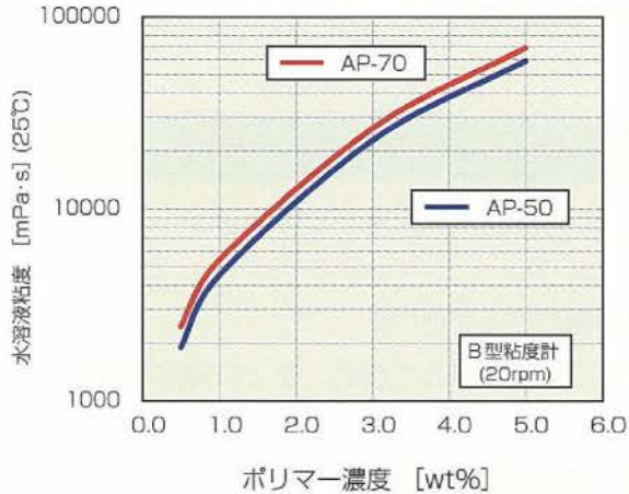
図1 水溶液濃度と粘度の関係
