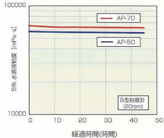
図3-2 40°Cでの5%水溶液粘度の経時変化
